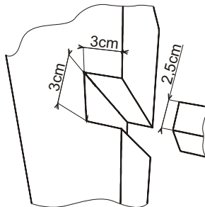
Obr. 1: Nákres zárezu do predného stĺpu zásobníka
